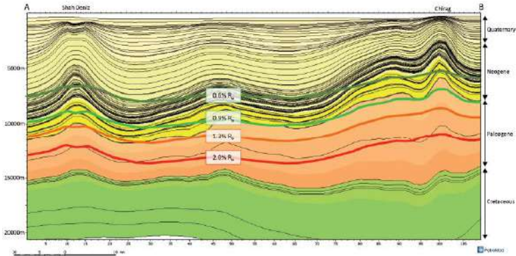
Şəkil 21. Stratiqrafik bölünməni və termal yetkinliyin izoxətlərini (EASY%Ro) nümayiş edən 3D modeli (Petromod paketi) əsasında regional profil. Hövzədəki karbohidrogenlərin yetkinliyini izah etmək üçün Şah-Dəniz yataq bölgəsindəki ana süxurlar 13 km-dən artıq olan dərinlikdə yerləşməlidirlər
