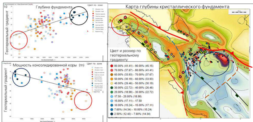
Şəkil 4. Geotermal qradiyentin yer qabığının və çöküntü örtüyünün qalınlığından asılılığı. Şəkilin sol tərəfindəki qrafiklər geotermal qradiyentin fundamentin dərinliyindən və konsolidasiya edilmiş qabığın qalınlığından asılılığını göstərir.
