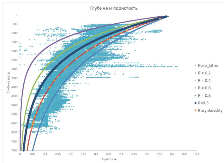
Şəkil 14. Hövzə boyu dərinlikdə çöküntülərin məsaməliliyinin və sıxlığının dəyişmə qrafiki. Karotaj məlumatları sıxılma ayriləri ilə əhatə olunur. Ən yaxşı korrelyasiya R=0,5 -dir.
